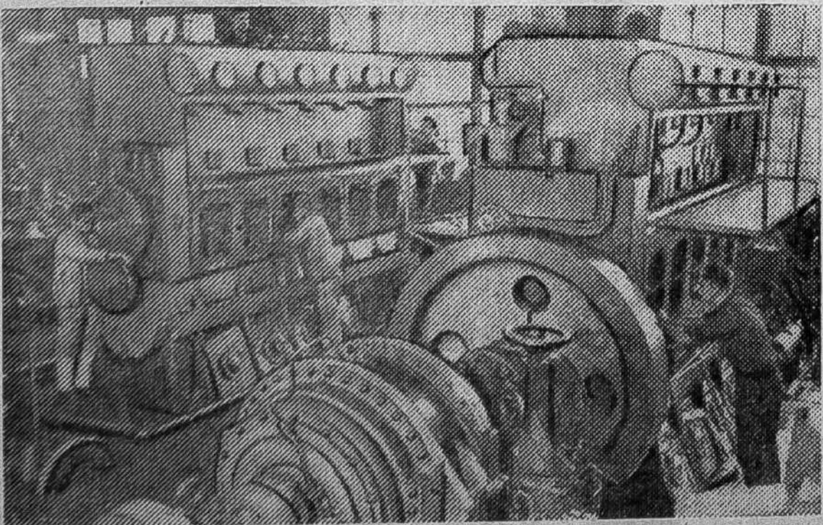
ГОРЬКОВСКИЙ дизельный завод «Двигатель революции» начал серийное производство дизелей мощностью в 900 лошадиных сил с газотурбинным наддувом. Отгружены первые машины предприятиям и стройкам. НА СНИМКЕ: сборка дизелей с газотурбинным наддувом мощностью 900 лошадиных сил. Фото Н. Акимова. Фотохроника ТАСС
