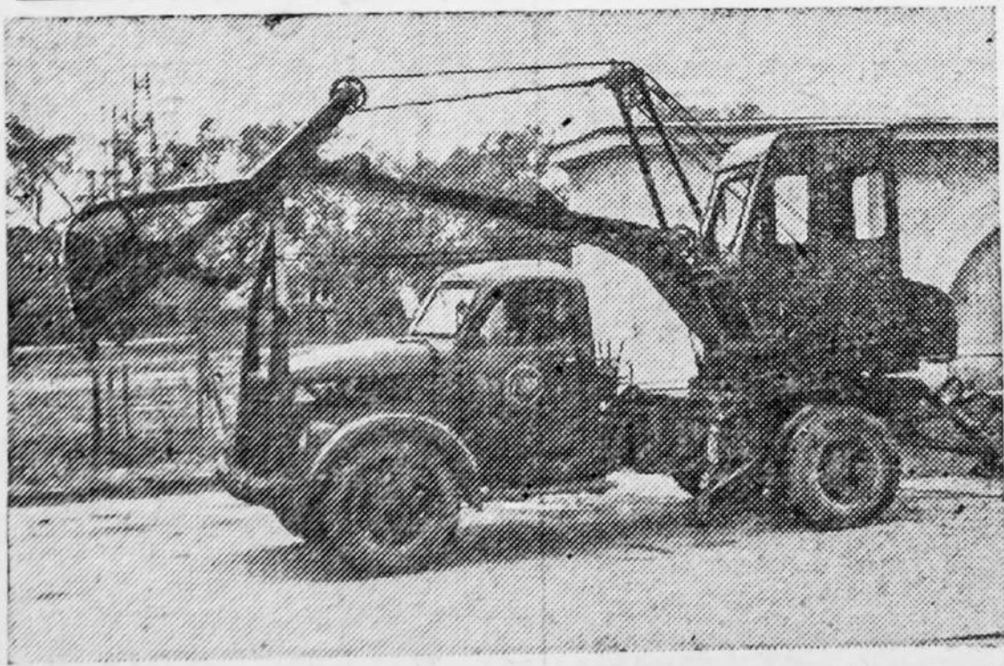
Ленинград. Специальное конструкторское бюро треста «Ленинградоргстрой» и Главленинградстрой разработало новый экскаватор на базе автомашины ГАЗ-51 с ковшем емкостью 0,15 кубических метра. Производительность его 50 кубических метров в смену. Предприятия Главленинградстрой приступили к выпуску таких машин.
