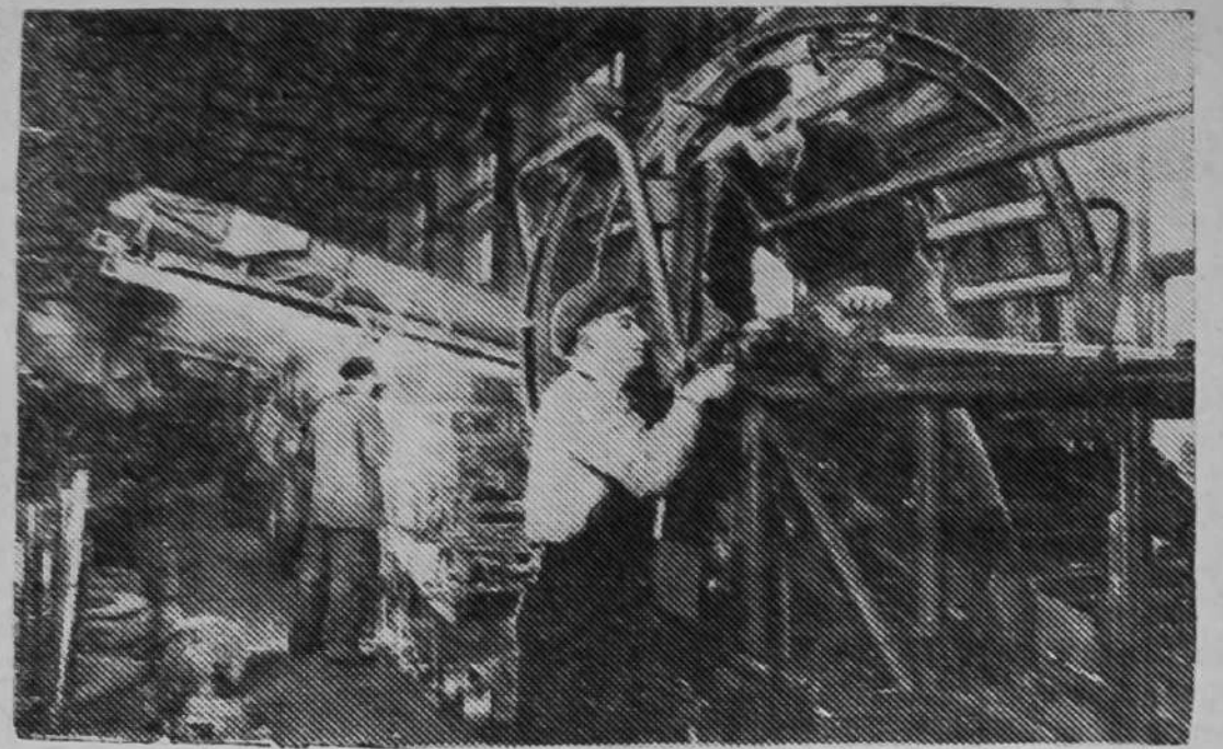
МОСКОВСКАЯ ОБЛАСТЬ. К выпуску новых картофелеуборочных комбайнов «КГП-2» приступил Коломенский тепловоозостроительный завод имени В. В. Куйбышева. В отличие от рязанского комбайна «ККР-2» новая машина более производительна и при уборке дает меньше потерь картофеля.
